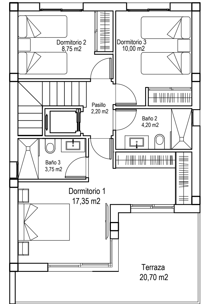
PLANTA PRIMERA
