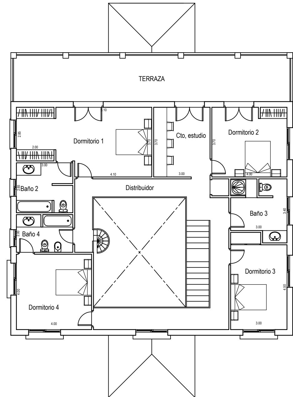
PLANTA PRIMERA
