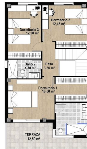
PLANTA PRIMERA
