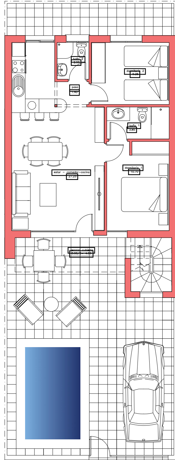
PLANTA BAJA
