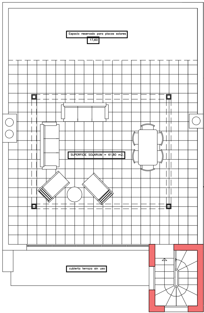
PLANTA SOLARIUM
