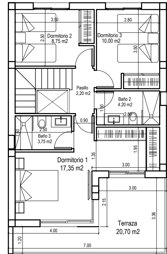
PLANTA PRIMERA
