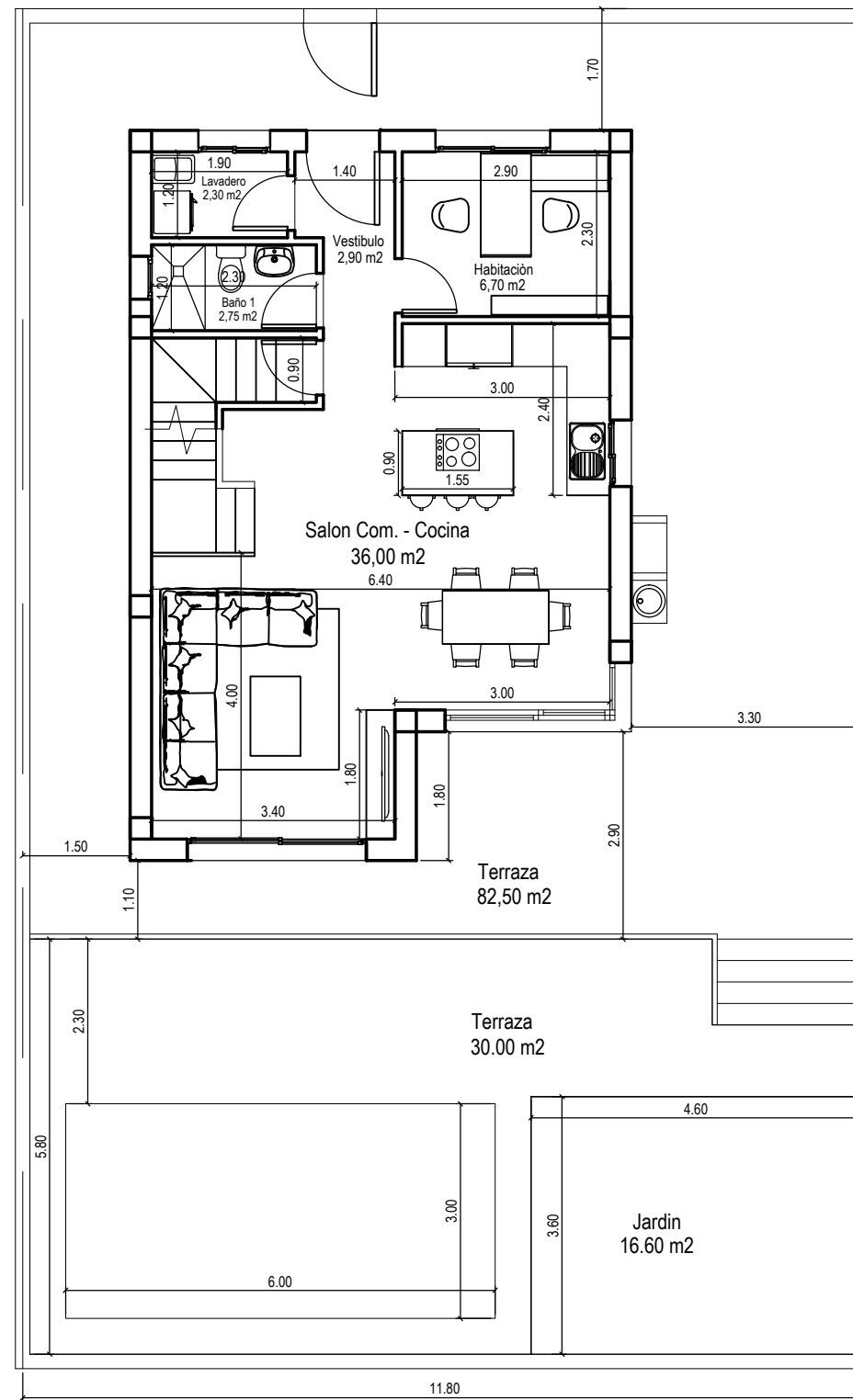
PLANTA BAJA
